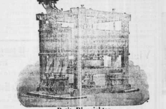
Petit Plansichter Le meilleur appareil de blutage pour petits moulins. — Grande production.
